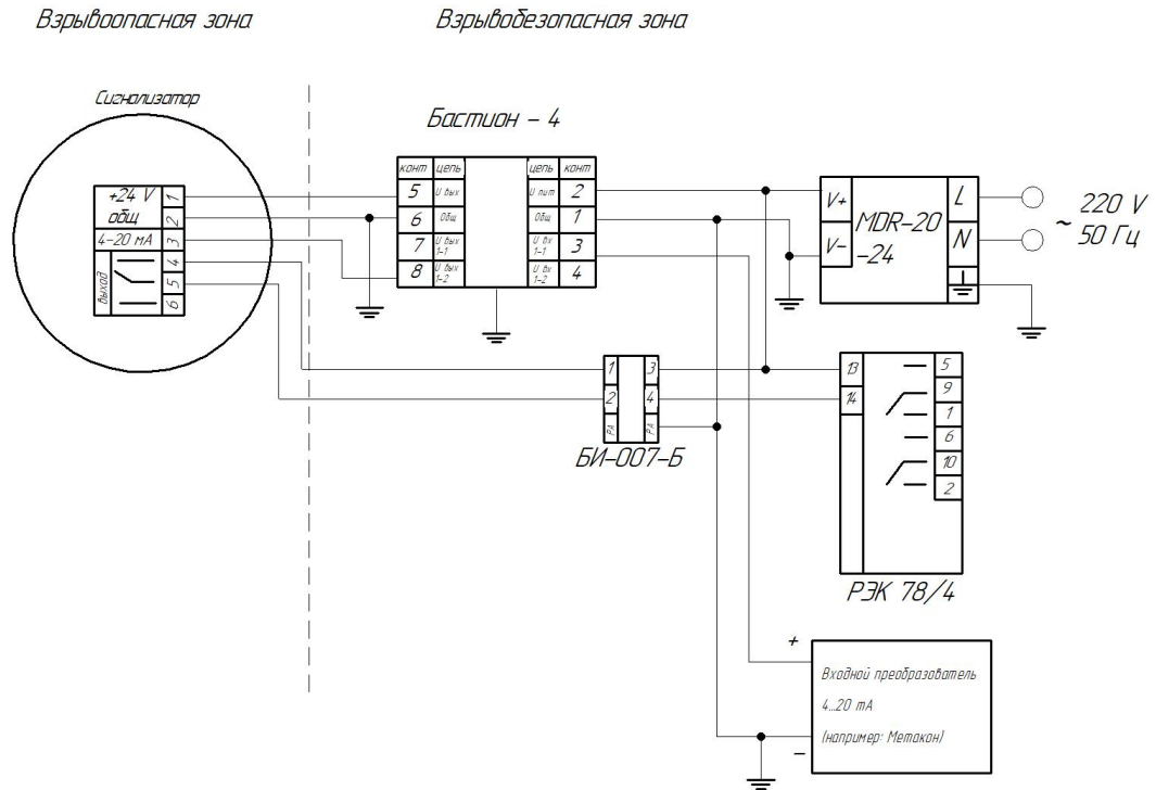
Рис. 7Б Подключение сигнализаторов с помощью барьеров искрозащиты с маркировкой взрывозащиты 0 Ex ia IС Т6 Ga X.
